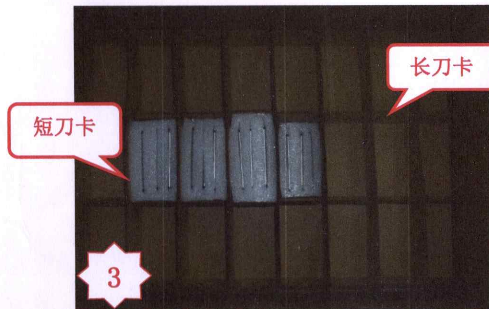
图三, 将 PA973 按照每格 6pcs, 每层 24 格, 每箱 3 层的方式包装, 同时在底部和每层的顶部各放一块隔板, 共 4 块隔板。
